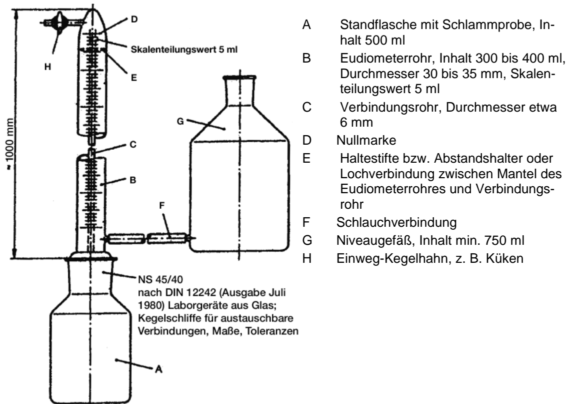
Bild 2: Versuchsanordnung zur Bestimmung des Faulverhaltens von Schlämmen nach DIN 38414-8, Seite 6, Ausgabe Juni 1985
