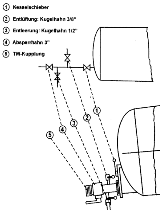
Probenahmeverrichtung an Vakuum-Tankwagen
