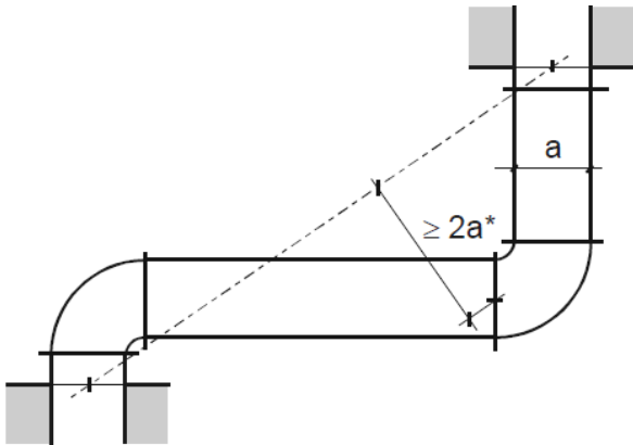
Bild 5.1: Begrenzung der Krafteinleitung mit Leitungsverziehung
