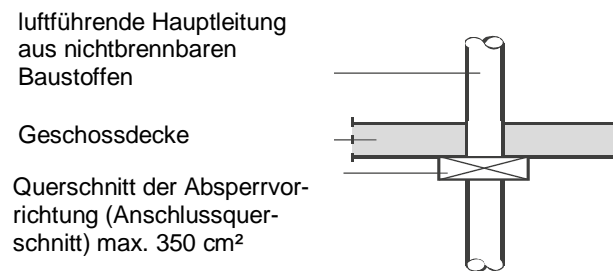
Bild 6.2: Beispiel für Schottlösung für Lüftungsanlagen nach DIN 18017 3:2009-09 maximaler Anschlussquerschnitt der Absperrvorrichtungen: 350 cm 2
