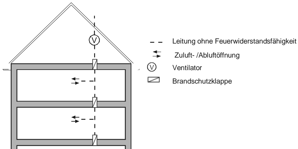
Bild 2.1: Schottlösung
