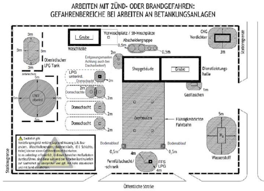
Abbildung 11: Arbeiten mit Zünd- oder Brandgefahren: Gefahrenbereiche bei Arbeiten an Betankungsanlagen
