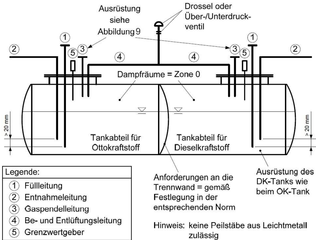
Abbildung 7: Ausrüstung von Lagertanks für Kraft- und Betriebsstoffe mit unterschiedlichen Gefahrenmerkmalen gemäß Abschnitt 2 Absatz 13 mit gemeinsamer Lüftungsleitung
