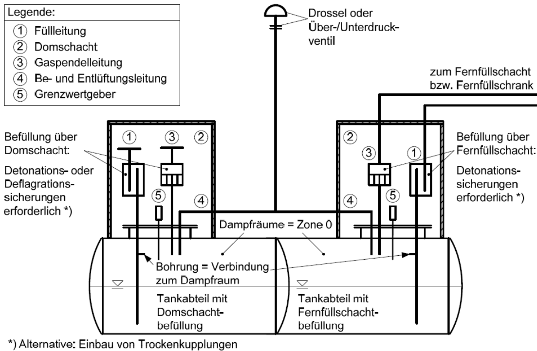
Abbildung 8: Flammendurchschlagsicherung an Lagertanks für Kraft- und Betriebsstoffe mit unterschiedlichen Gefahrenmerkmalen gemäß Abschnitt 2 Absatz 13 mit gemeinsamer Lüftungsleitung
