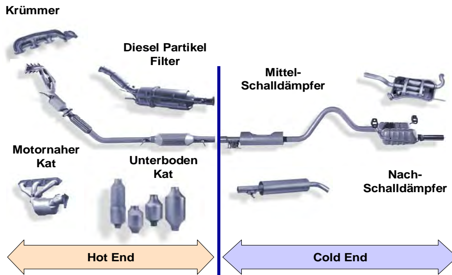
Hot-End und Cold-End einer Abgasanlage
