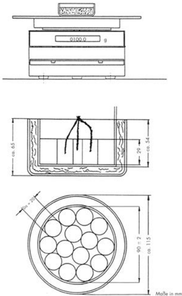
Abbildung 4: Prüfung der Abbrandgeschwindigkeit von flüssigen organischen Peroxiden
