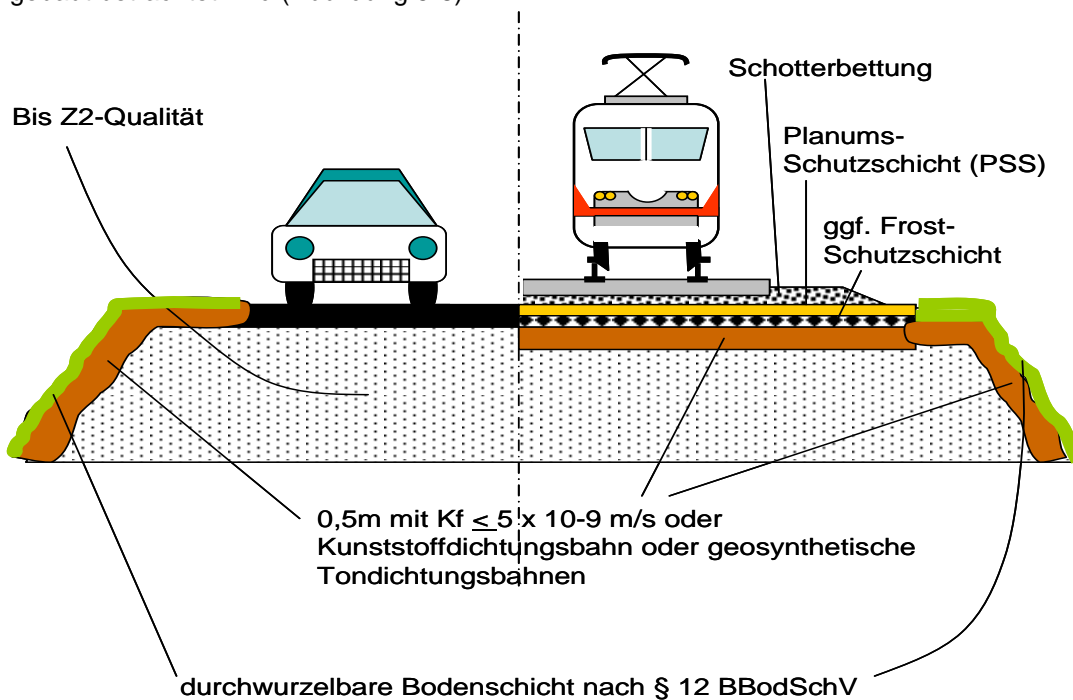
Abbildung 5-7 Regelbauweise Verkehrswegedamm
