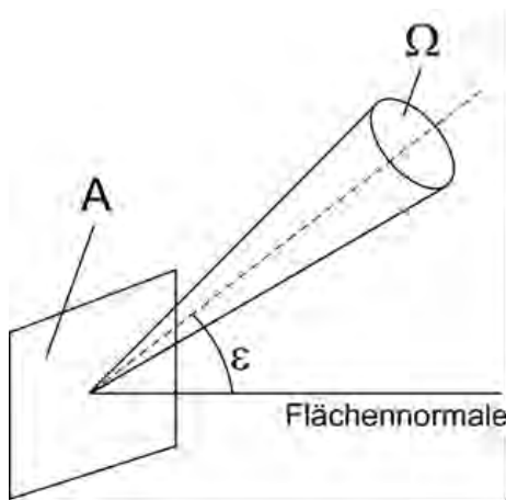
Abb. 2 Strahldichte L unter einem Winkel \varepsilon
