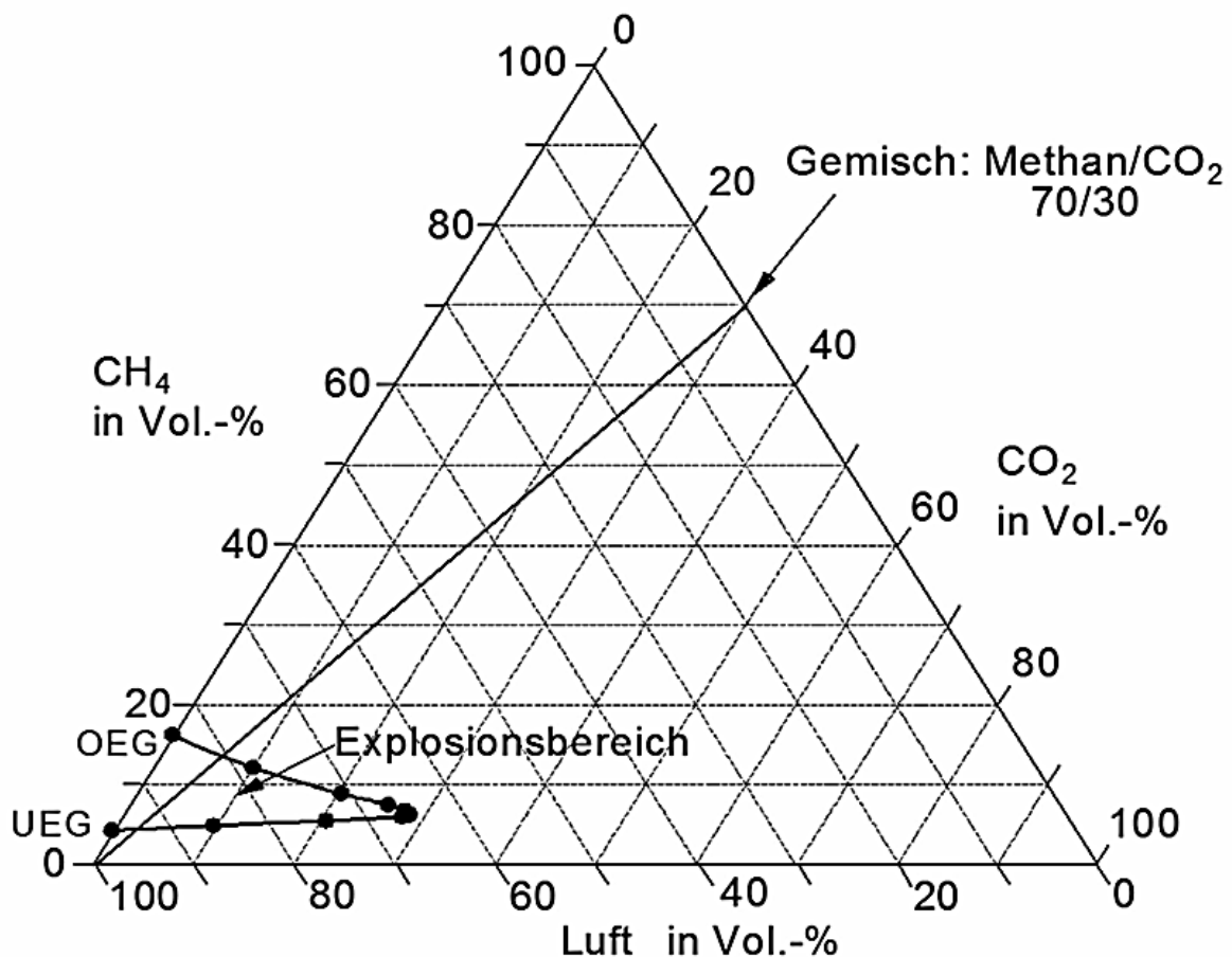
Abbildung 1: Explosionsbereich von Methan-Kohlendioxid-Gemischen - Dreiecksdiagramm, /16/
