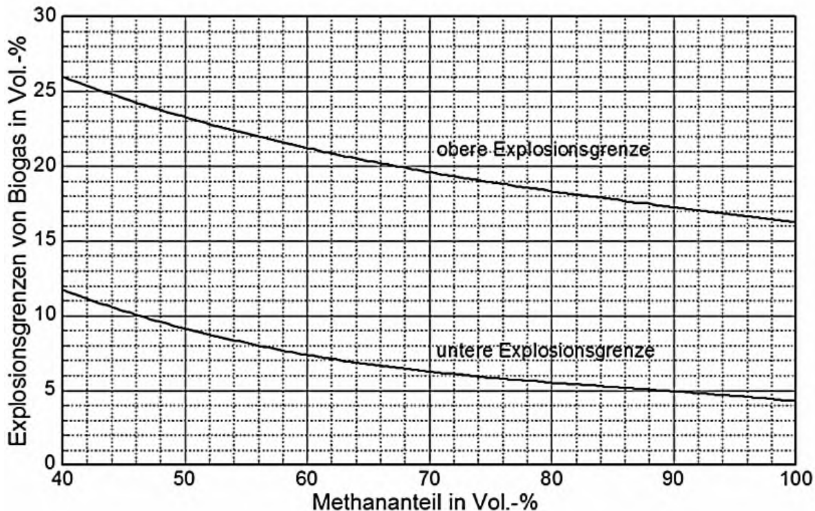
Abbildung 2: Explosionsgrenzen von Biogas in Abhängigkeit vom Methananteil /16/
